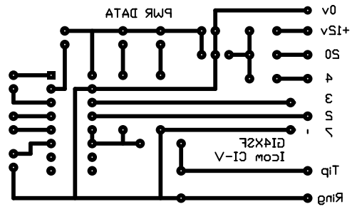
ICOM4 Top Layer
